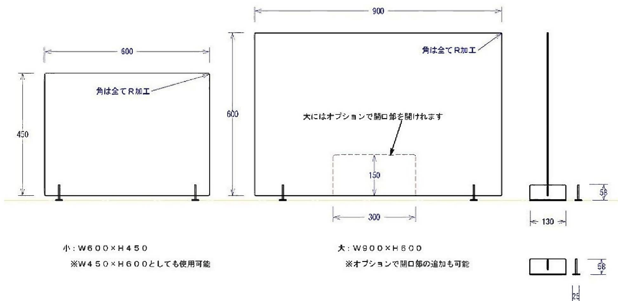
アクリル透明仕切り板 新型コロナウイルス対策用 飛沫感染防止
